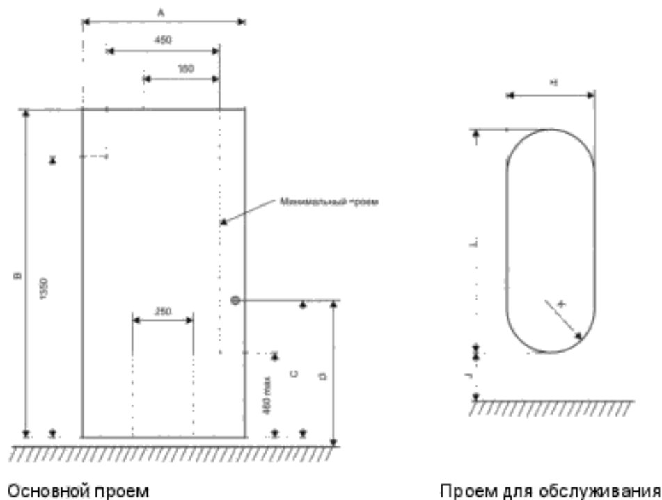
Рисунок 1 – Проемы
