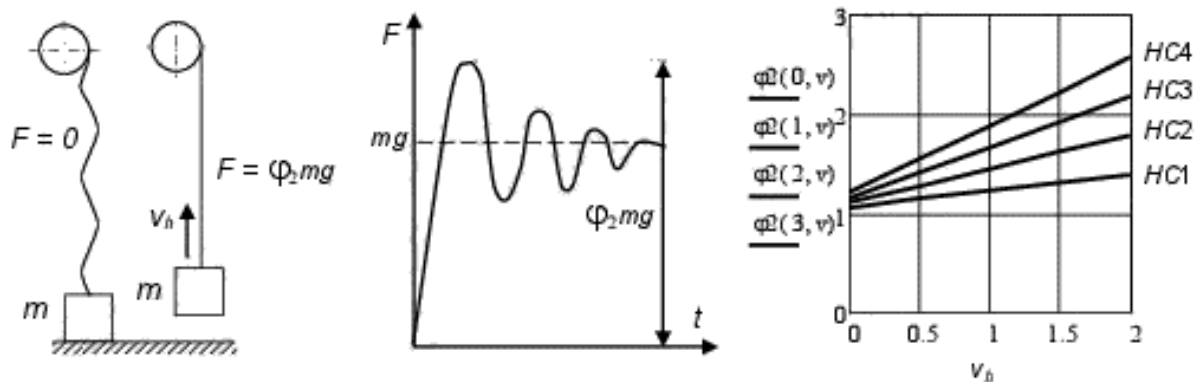
Рисунок 1 – Схемы к определению коэффициента \varphi_2
