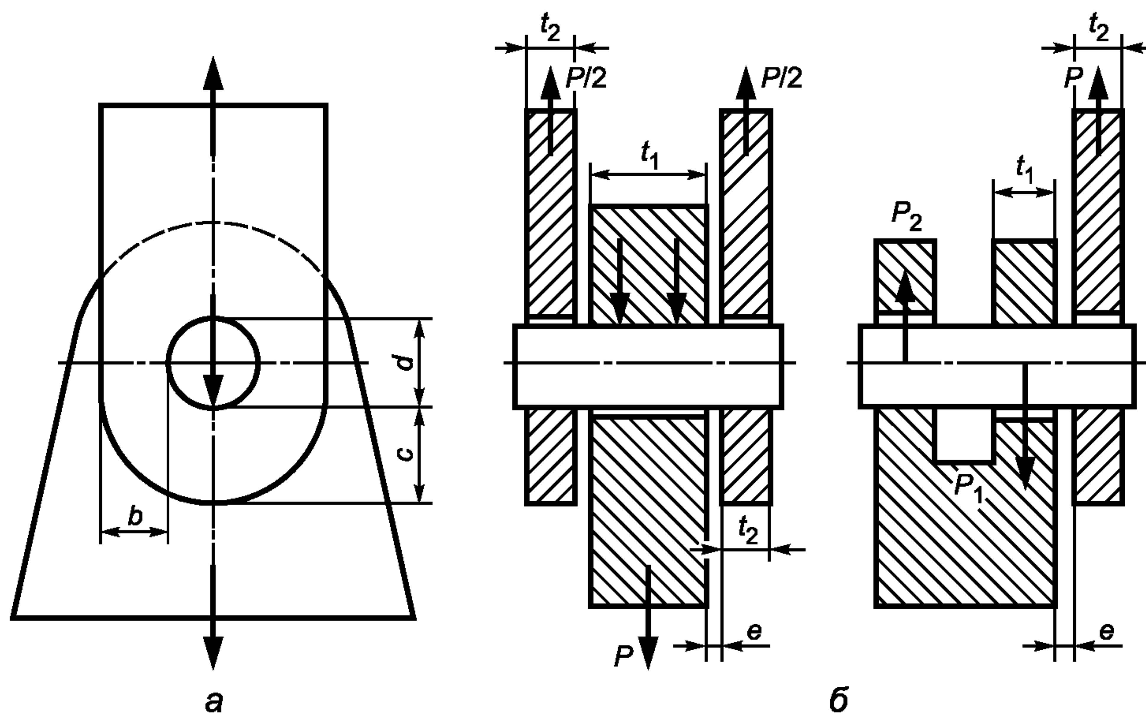
Рисунок 10 — Схема шарнира с проушиной
