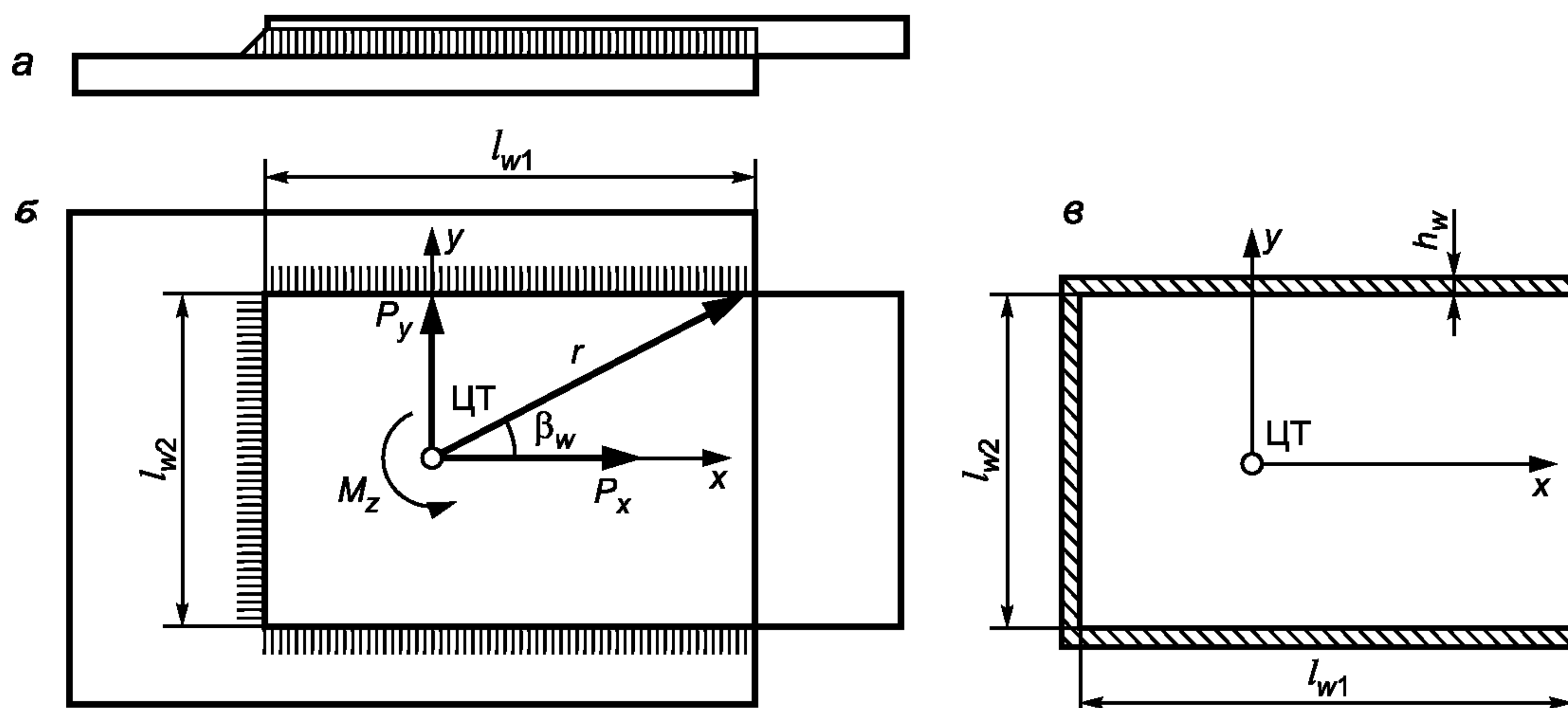
Рисунок 4 — Схема сварного нахлесточного соединения ( a ) и площадь среза шва ( б )
