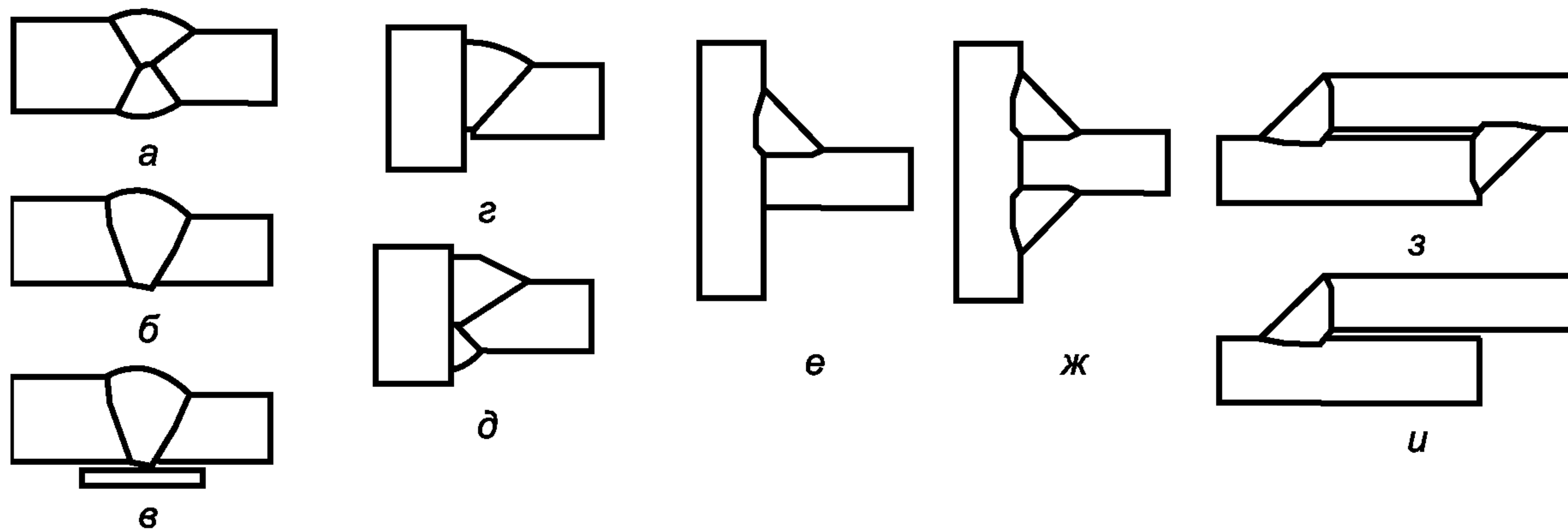
Рисунок 2 — Схемы сварных соединений
