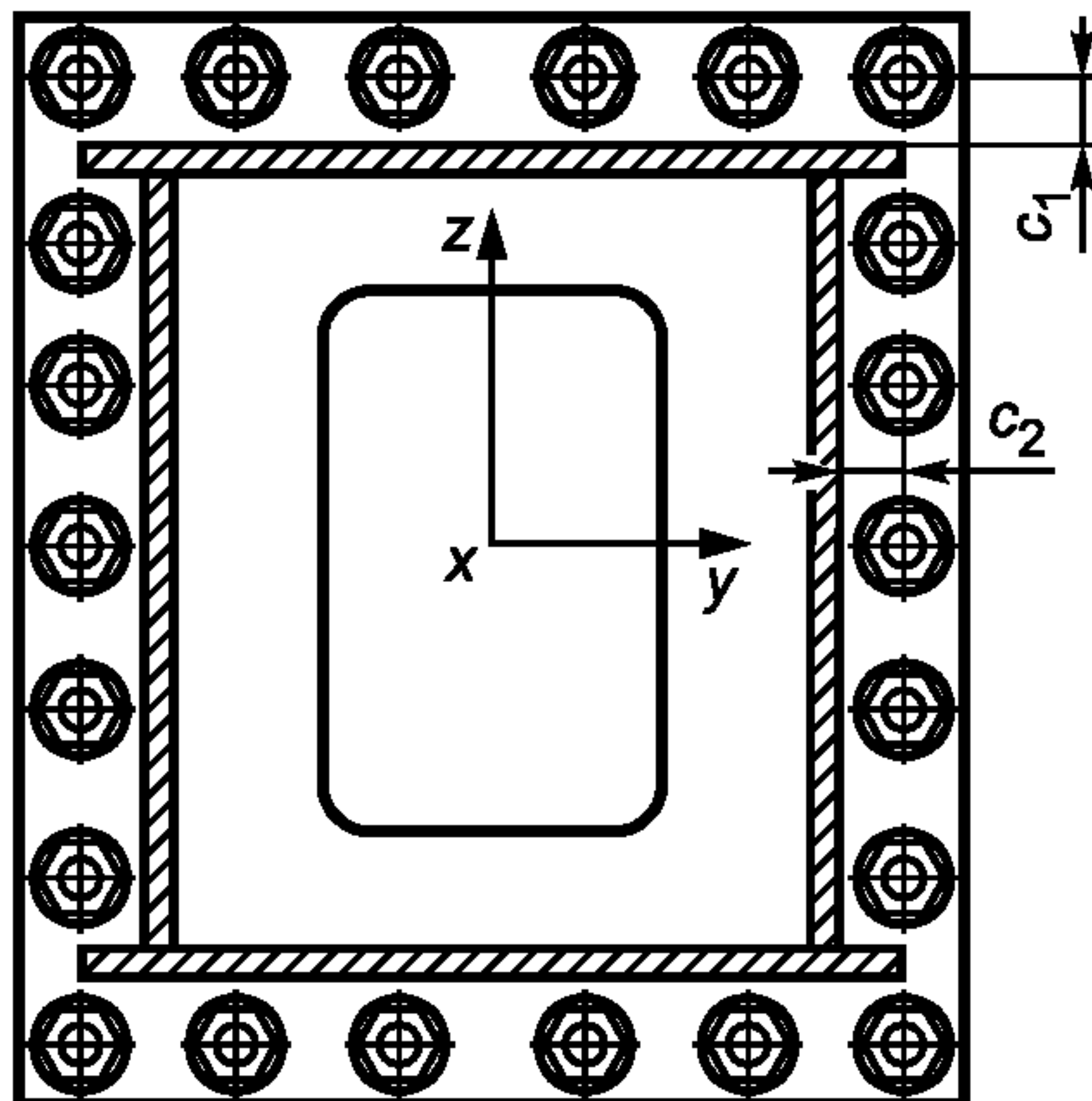
Рисунок 6 — Пример схемы размещения болтов во фланцевом соединении
