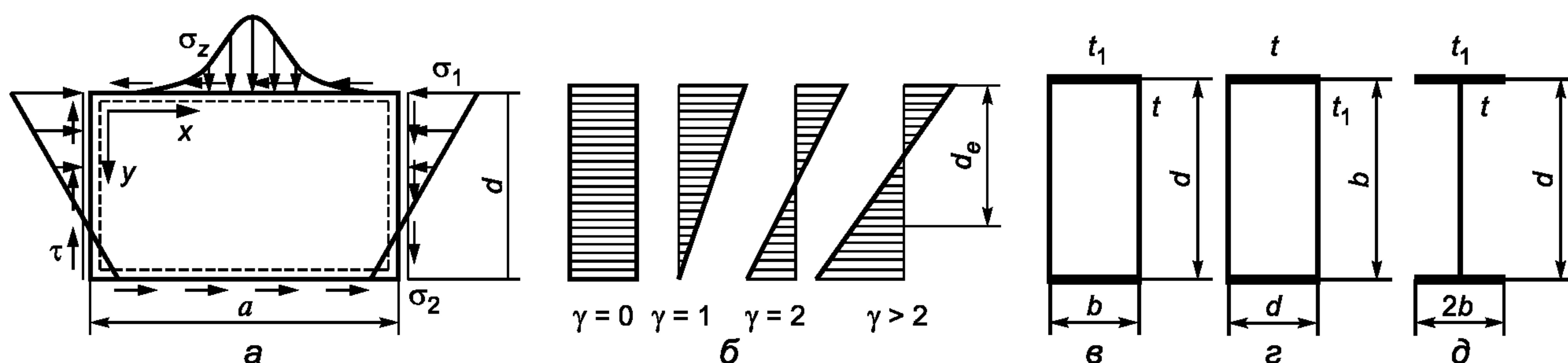
а — общий случай нагружения пластины; б — эпюры распределения нормальных напряжений \sigma ; в, г, д — обозначения расчетных размеров пластин для расчета стенки коробчатой балки, пояса коробчатой балки и стенки двутавровой балки.
