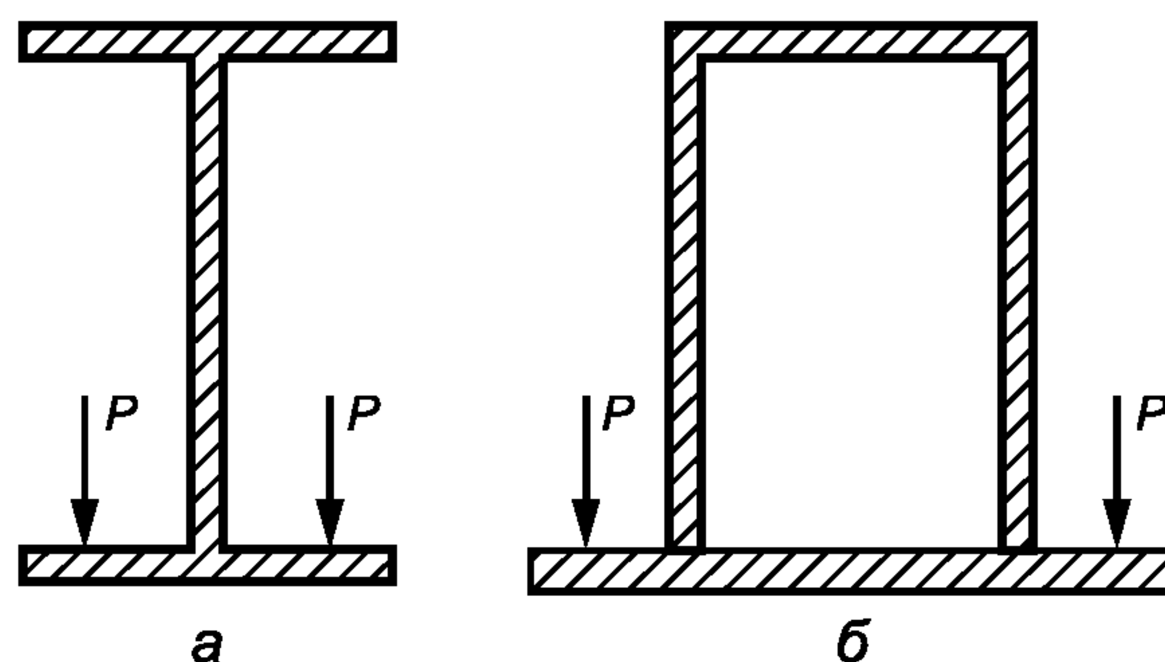
Рисунок А.2 — Схемы ездовых балок
