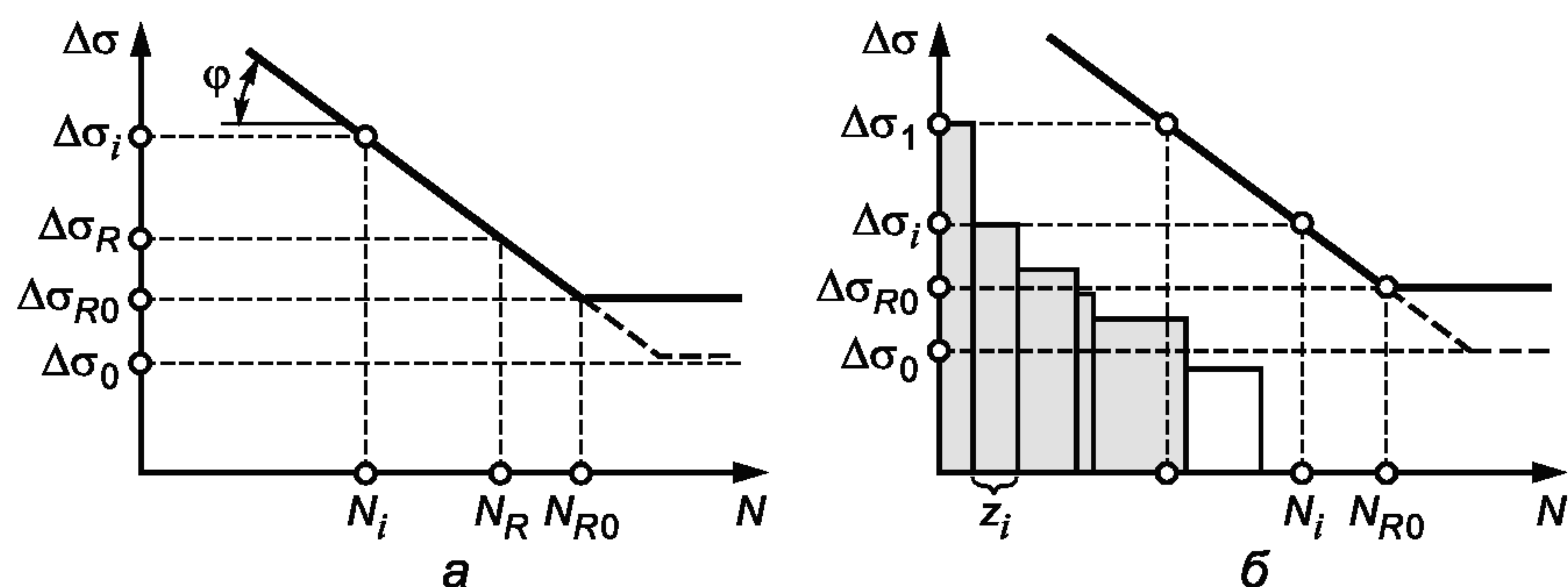
Рисунок 15 — Схемы усталостной кривой, построенной в логарифмических координатах
