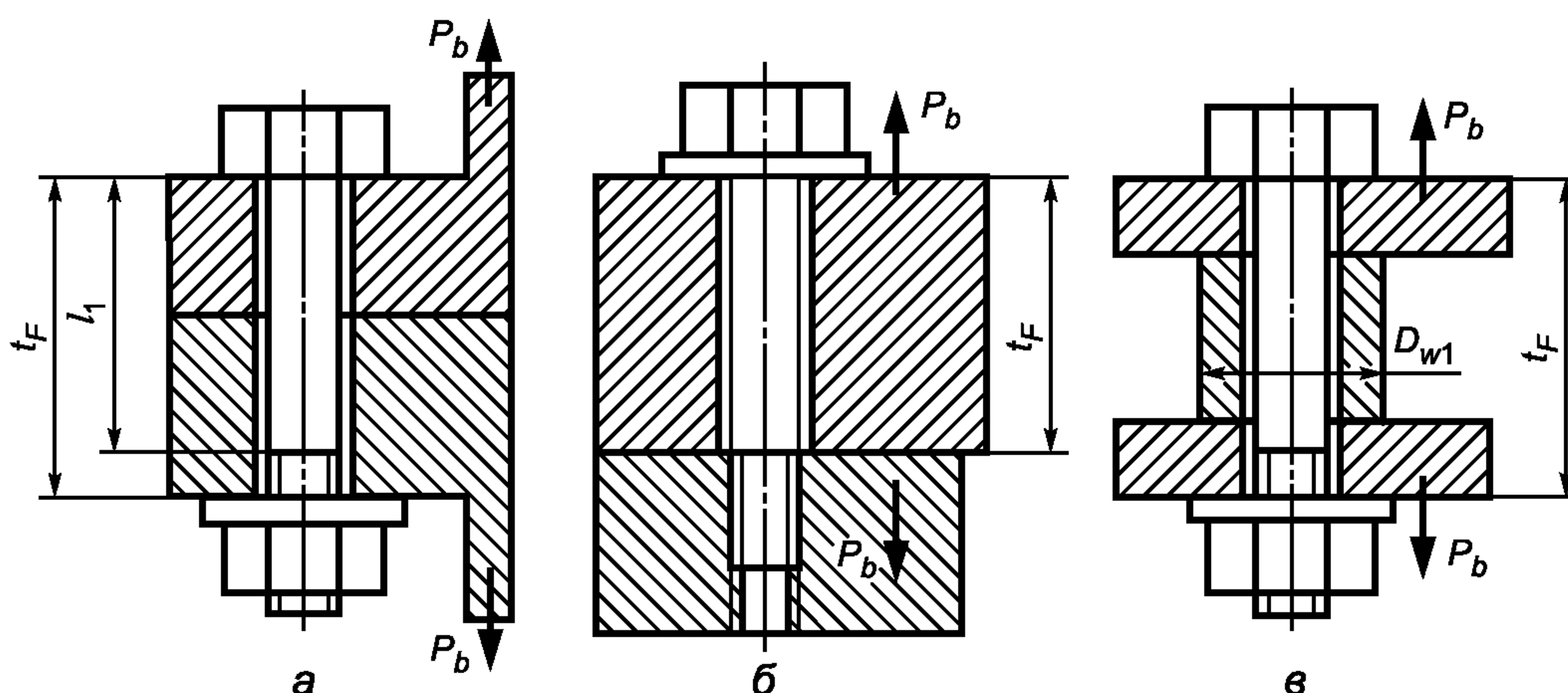
Рисунок 7 — Схемы установки болтов во фланцевом соединении
