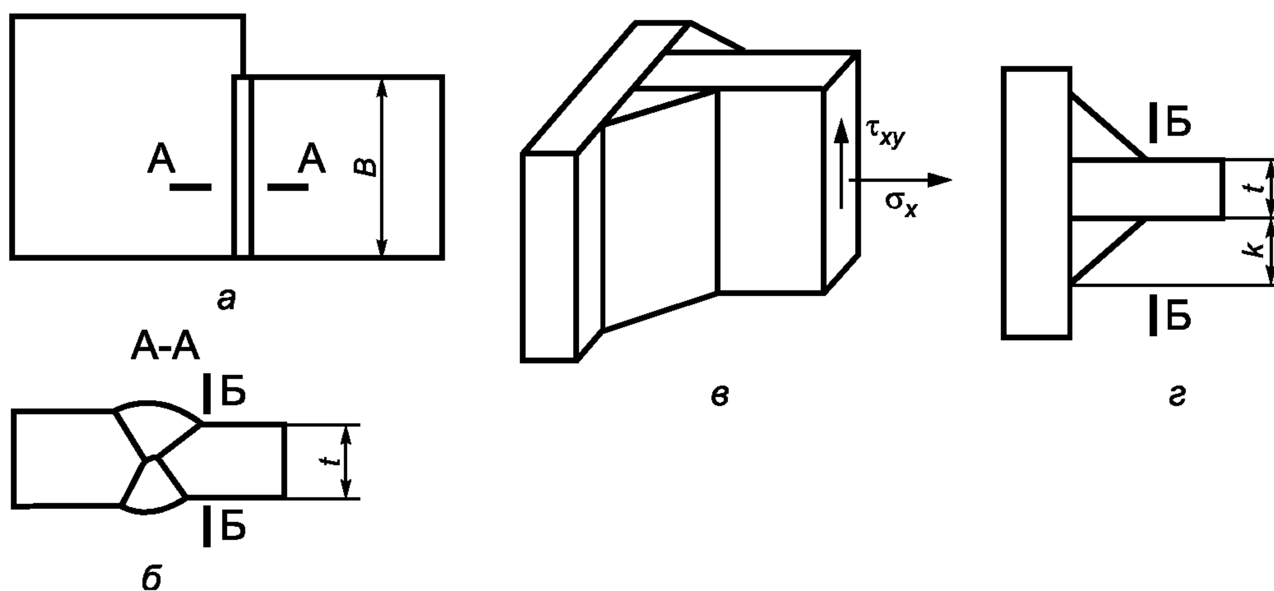
Рисунок 3 — Схемы сварных соединений
