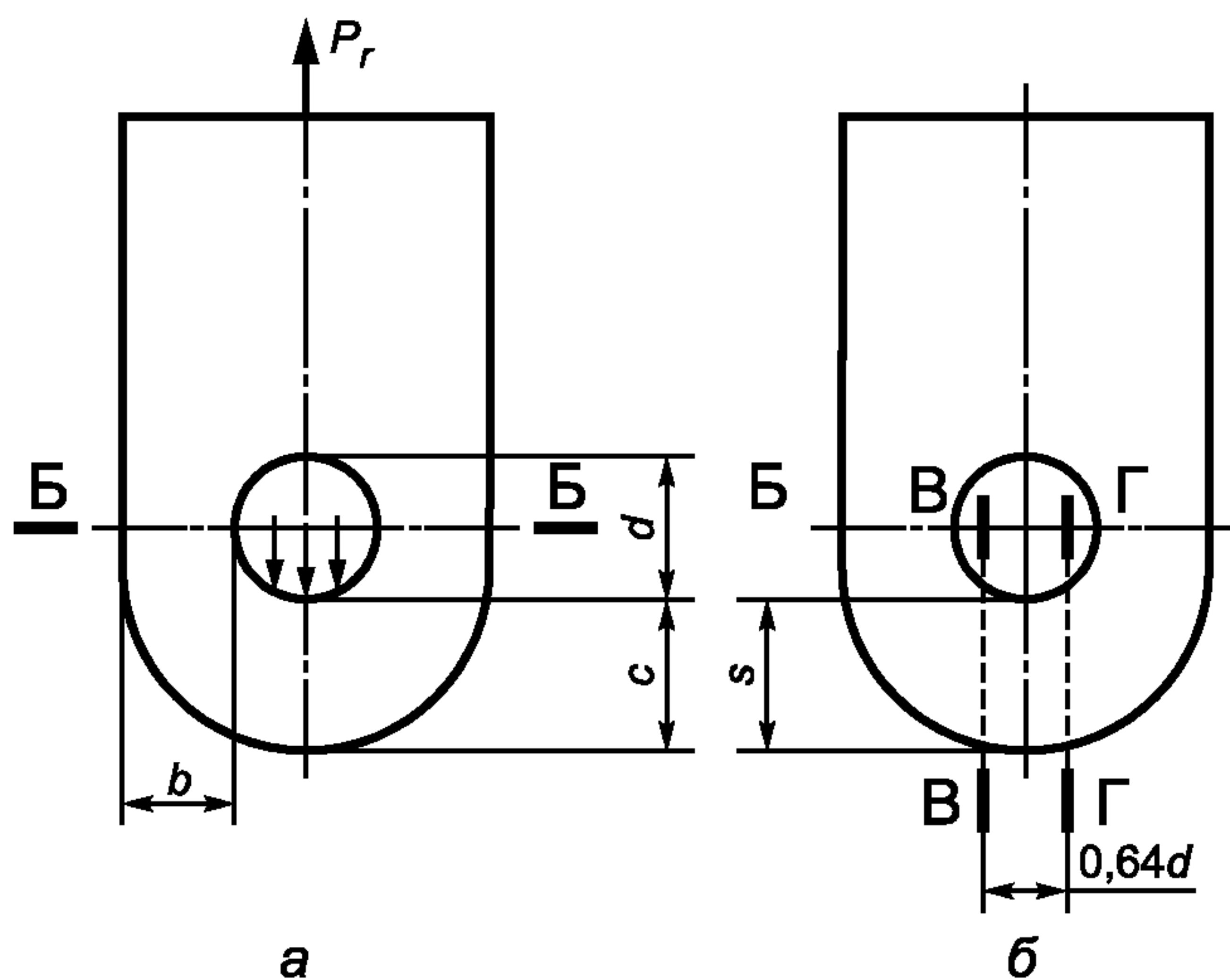
Рисунок В.1 — Схема проушины
