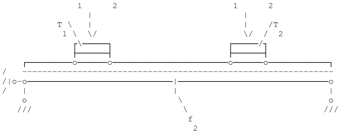
Рис. 7.3. Схема к проведению статических испытаний кранов с двумя грузовыми тележками на одних пролетных балках: а - п. 1.2.1; б - п. 1.2.2, б; в - п. 1.2.3
