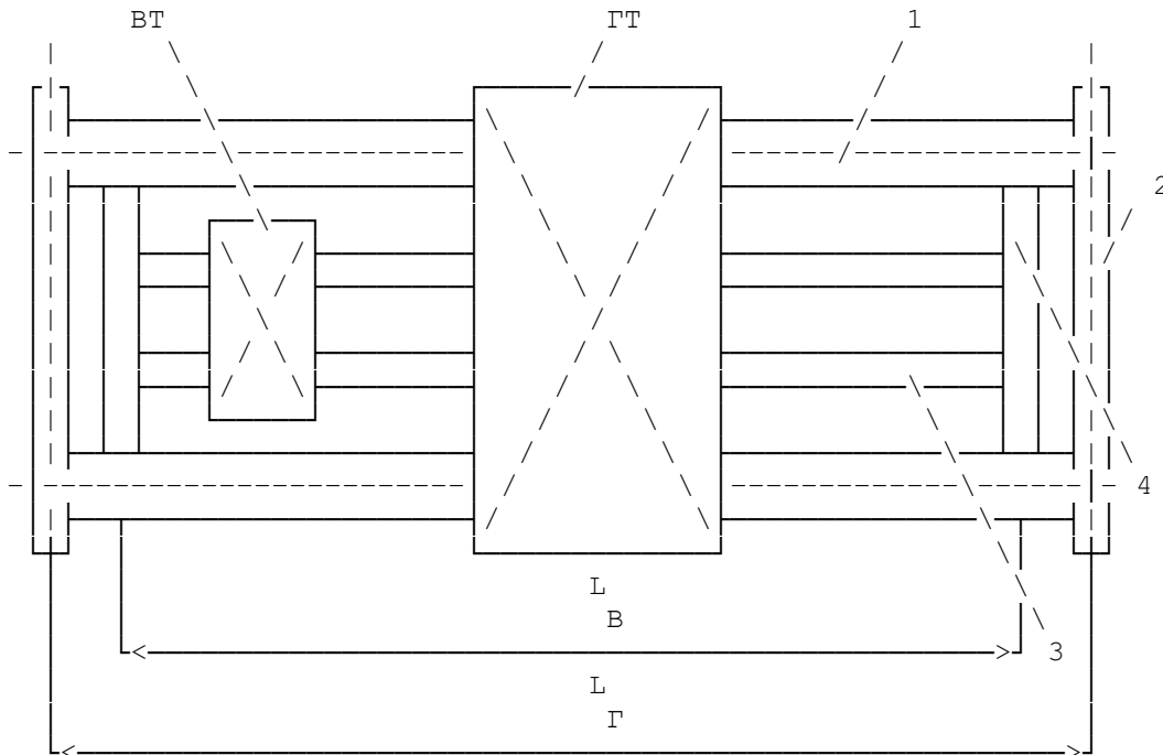
Рис. 7.4. Схема моста литейного крана: ГТ - главная тележка; ВТ - вспомогательная тележка; 1 - пролетная балка главного моста; 2 - концевая балка главного моста;
