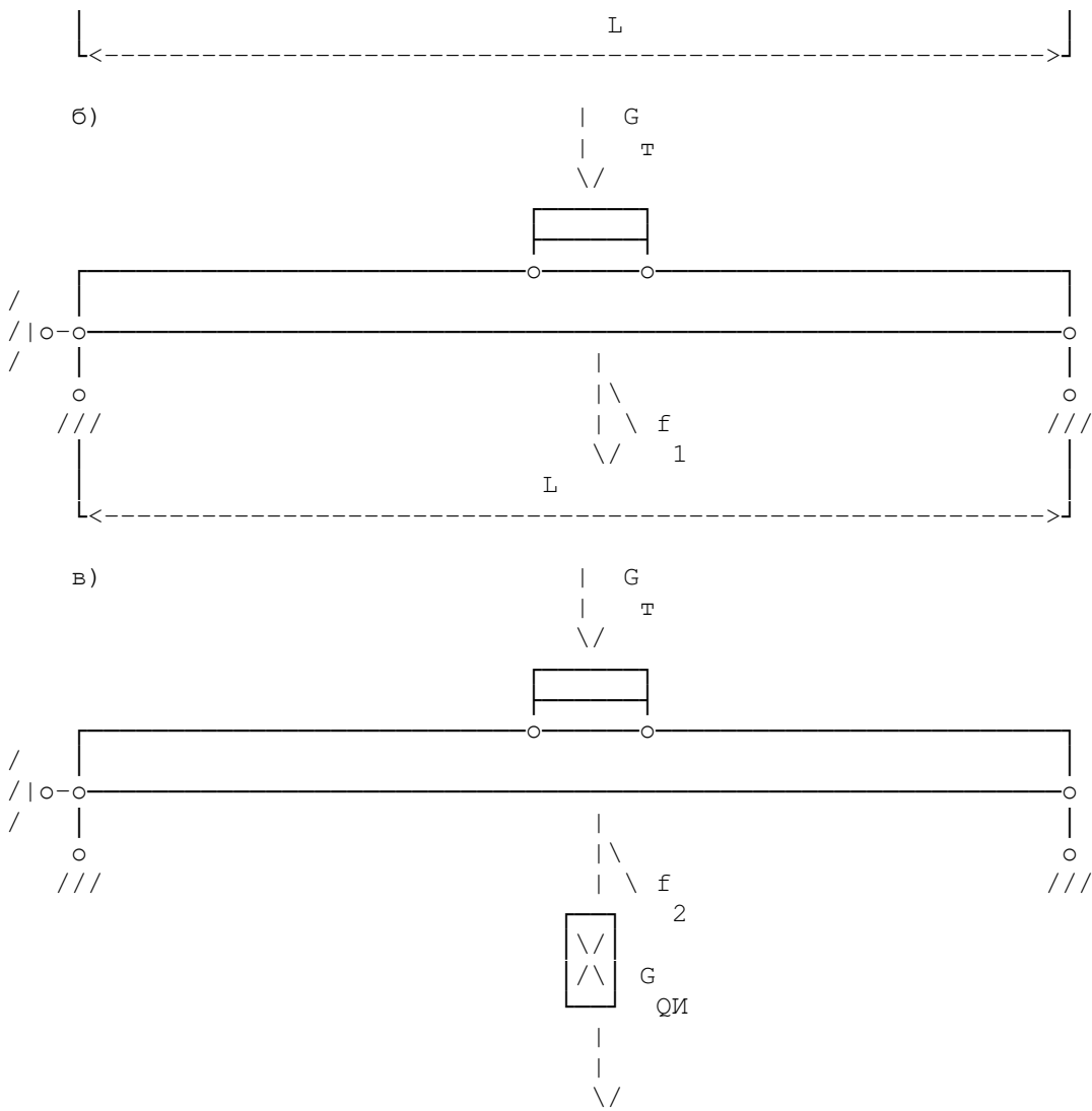
Рис. 7.1. Схемы к проведению статических грузовых испытаний кранов с одной тележкой
